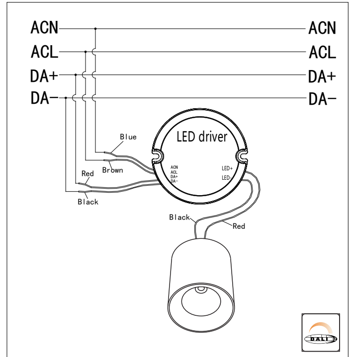
DALI Wiring
