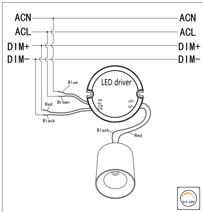
0/1-10V Wiring
